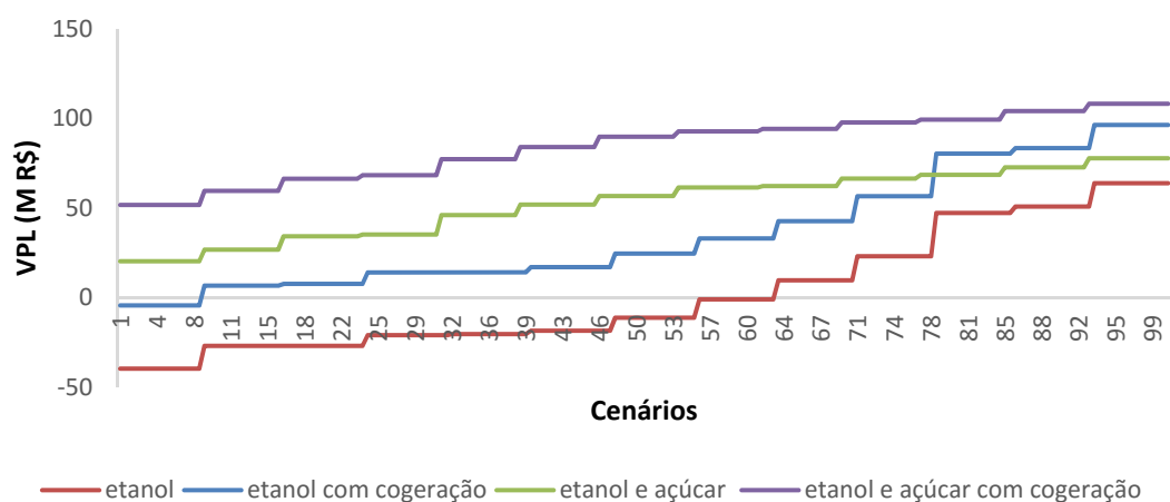
Figura 12 - VPL por cenário - Etanol esperado
