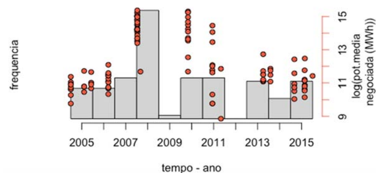
Figura 2 - Frequência de leilões cujo combustível é cana-de-açúcar e potência média negociada por usina entre 2005 e 2015 (em log(MWh))
