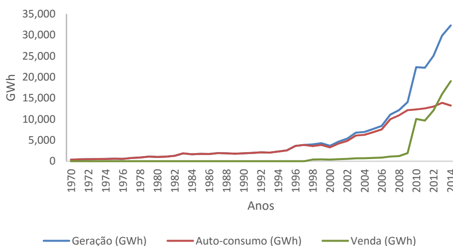
Figura 1 - Geração total versus Energia injetada no SIN entre 1970 e 2014 (GWh).
