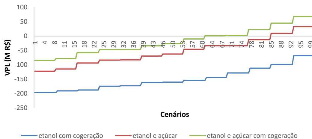
Figura 13 - VPL por cenário - Etanol observado
